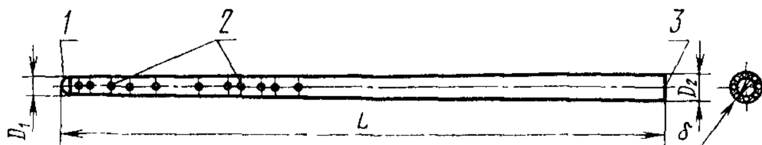
1—заглушка верхняя; 2—отверстия для крепления траверс; 3—заглушка нижняя.
